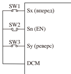
Рисунок 19, 3-проводное управление 1
